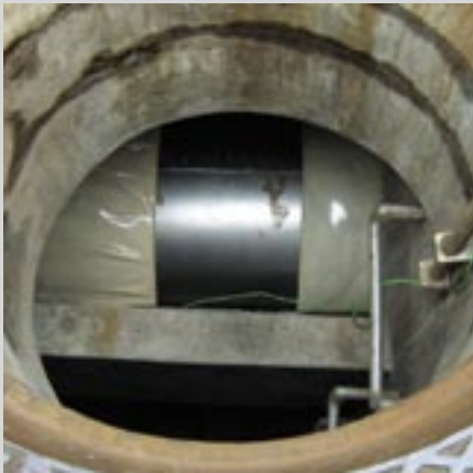
Entnahme Probekörper
